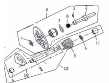
SISTEMA ARRANQUE (por patada)
